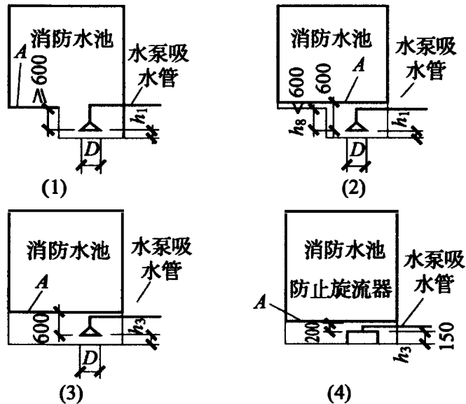
图2 消防水池最低水位
