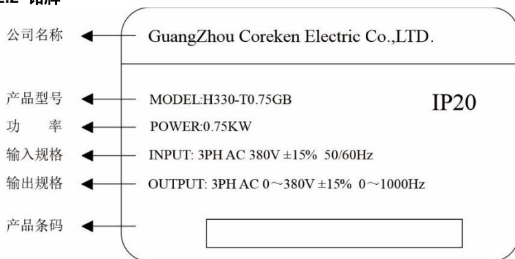
图 2-2 铭牌
