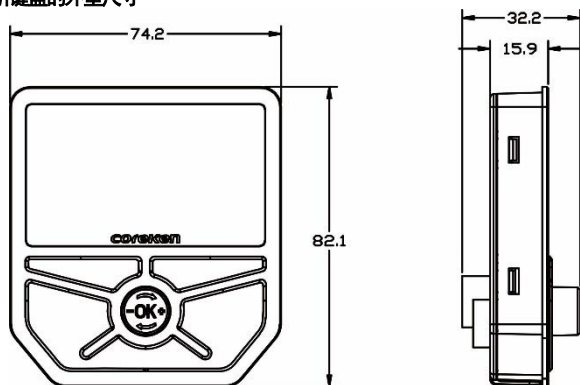
图 2-5 外引键盘的外型尺寸(单位: mm)
