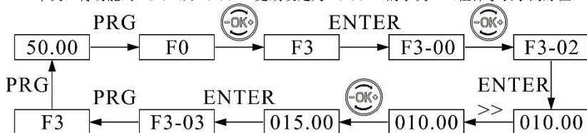
图 4-3 三级菜单操作流程 2
