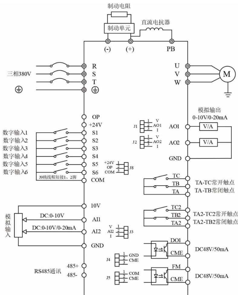
图 3-3 30~400kW 变频器接线示意图
